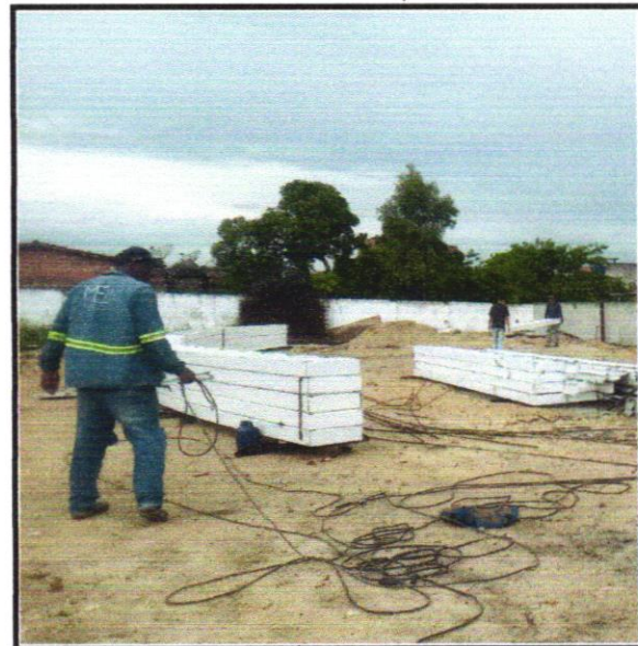
FOTO - 04: ESTRUTURA TRELIÇADA DE COBERTURA;
