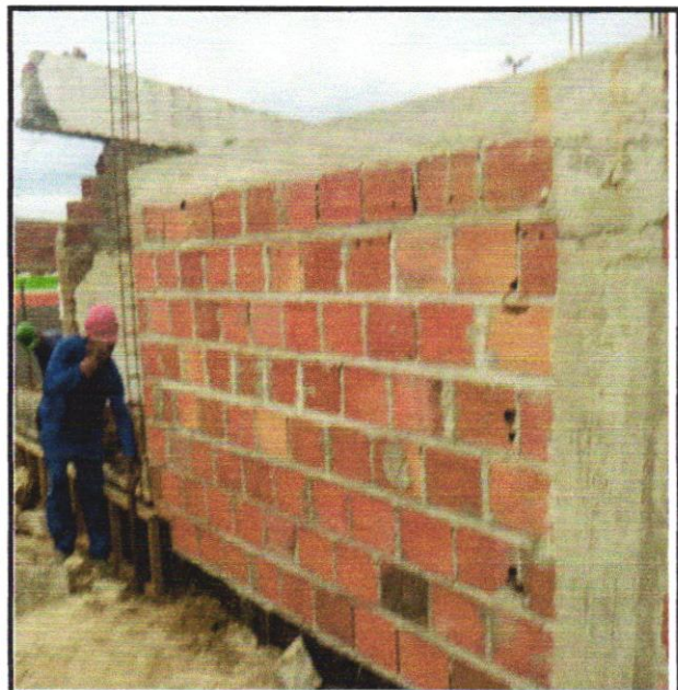
FOTO- 24 ALVENARIA DE VEDAÇÃO DE BLOCOS CERÂMICOS FURADOS NA HORIZONTAL DE 9X19X19
